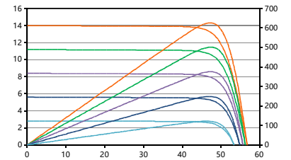
功率-电压&电流-电压曲线
