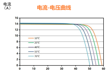
电流-电压曲线
